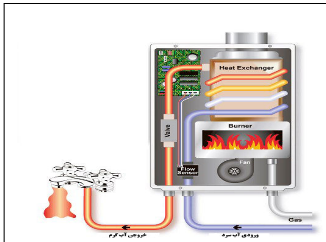
نحوه کارکرد آبگرمکن
